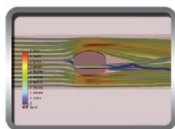
风动导流拍框 直观的看到有空气从导风槽 中流过, 卓越降低风阻
